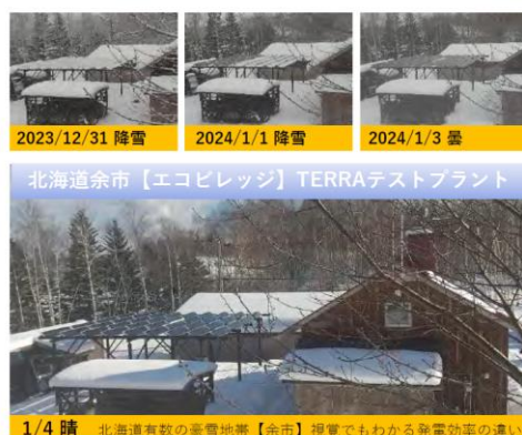
図 7 北海道での細型パネル太陽光発電のテストプラント 出所:株式会社 TERRA
